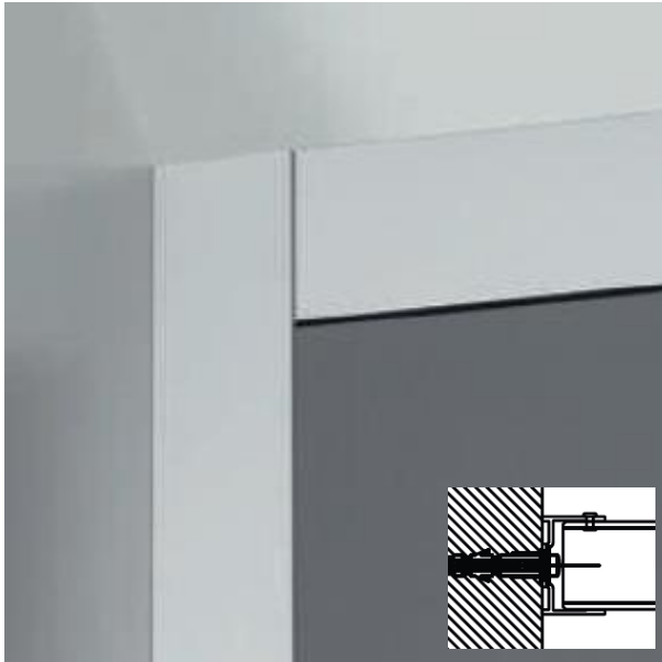
raccordo a muro con profilo a U per la compensazione di eventuali tolleranze
